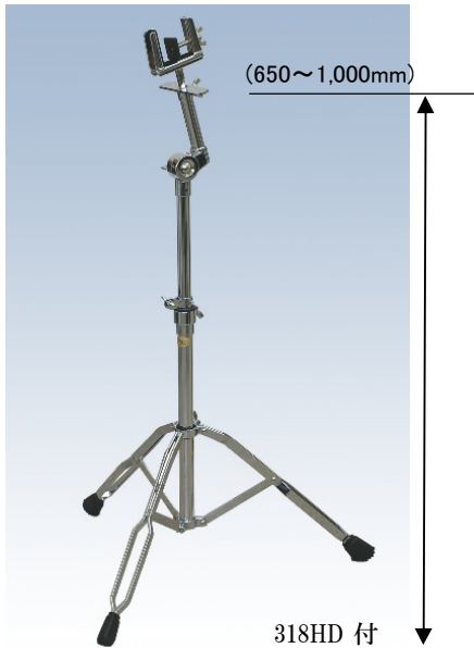
318NDX ホンゴスタンド ¥14,000 角度調節可能(三脚Wタイプ) 高さ調整(ホンゴ本体底部まで) 650mm ~ 1,100mm
