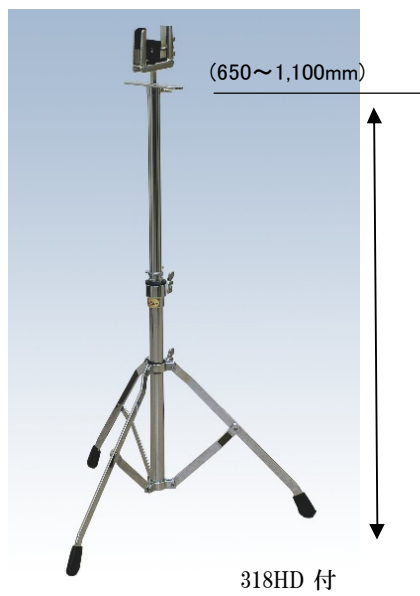
318 ホンゴスタンド ¥13,000 ストレートタイプ(三脚シングルタイプ) 高さ調整(ホンゴ本体底部まで) 650mm ~ 1,000mm
